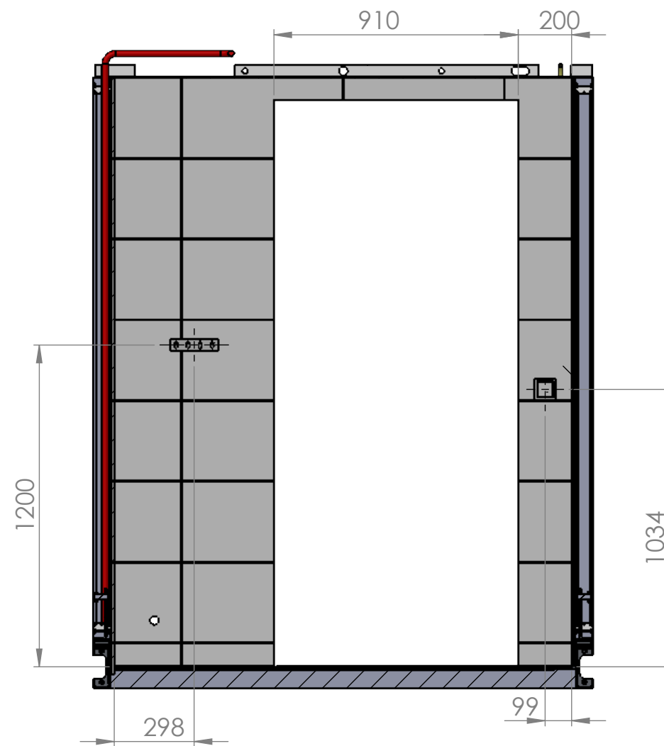
SECTION N-N SCALE 1 : 20
